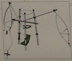
CANOPUS
